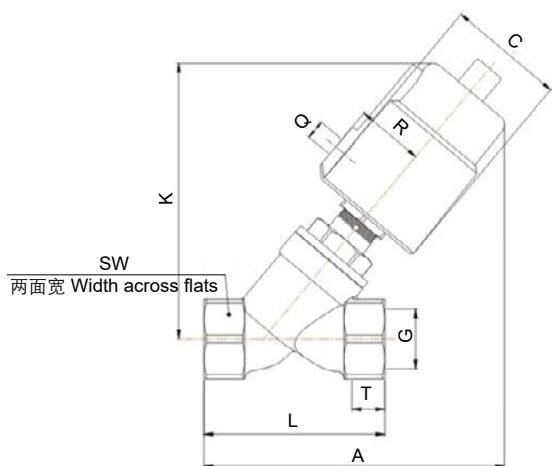
螺纹连接式 Threaded Connection
