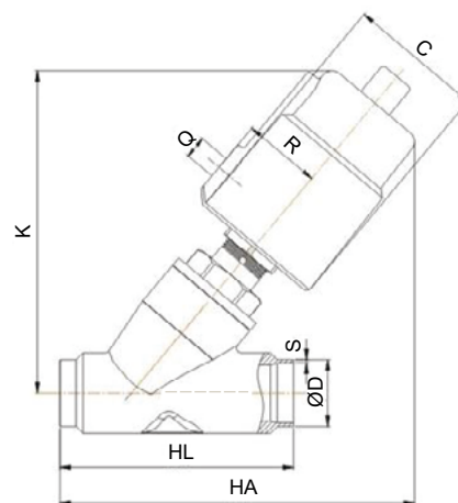
焊接连接式 Welded Connection
