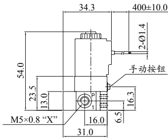
KSV211-G 常闭
