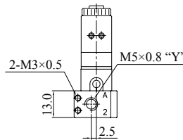
KSV212-G 常开
